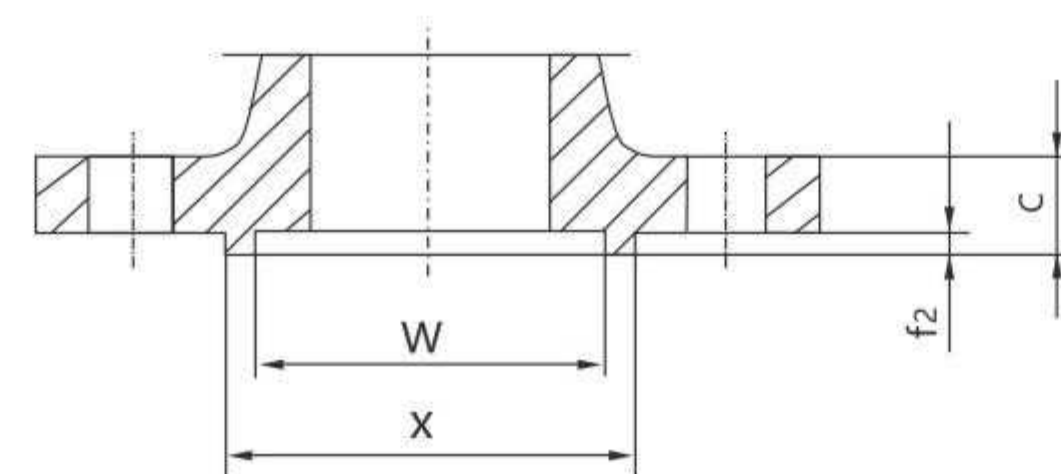
榫面 (T)
