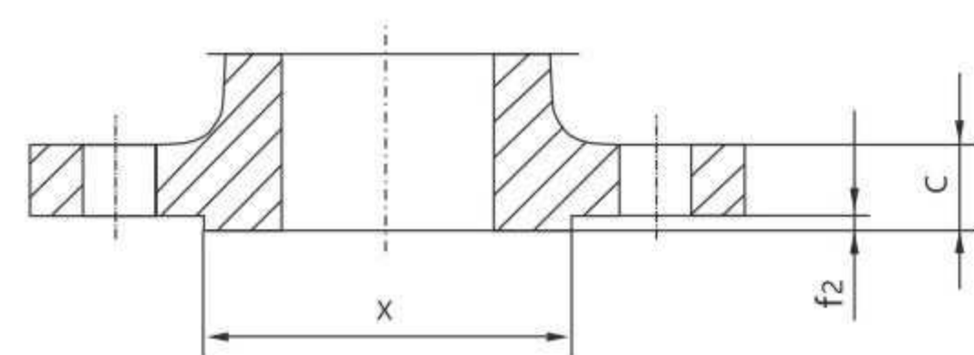
凸面 (M)
