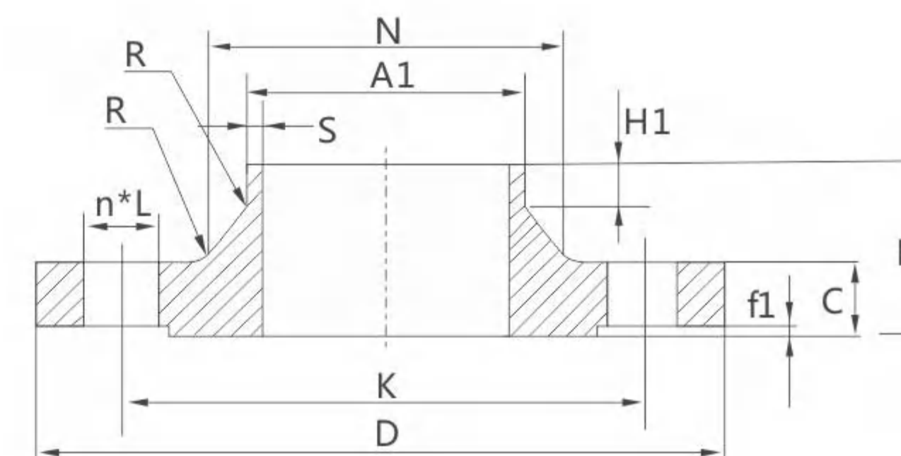
PN10带颈对焊钢制管法兰
