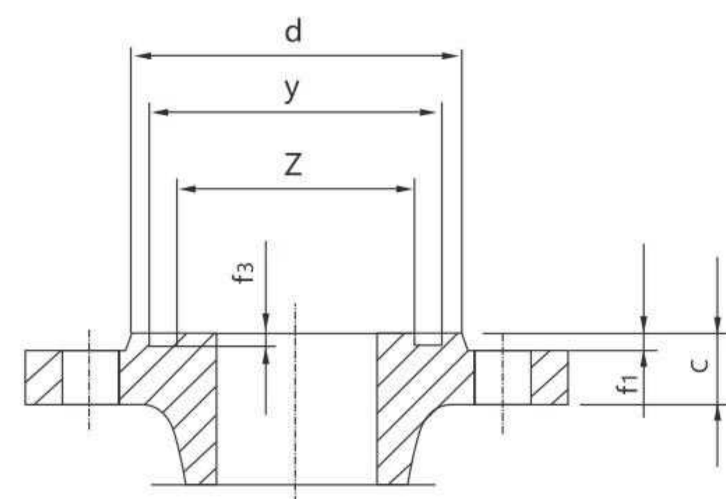
槽面 (G)
