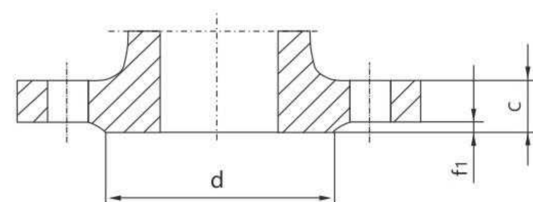
突面 (RF)
